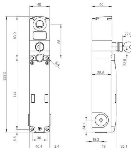
Switch NG 2D5D●●1 A
