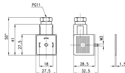
Габаритні розміри
