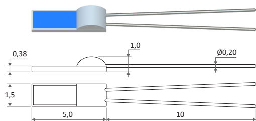
Платиновий резистор PCA 1.1505
