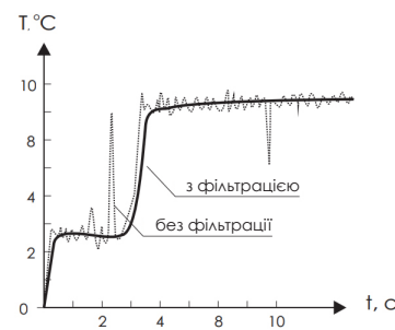
Рис. 3 Програмна фільтрація перешкод і нестабільності показань
