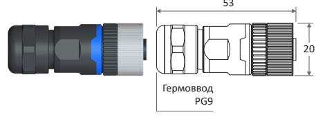
Роз'єм M12FD
