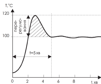
Стандартний ПІД регулятор (налаштування, паяльник, T_z=100^\circ\text{C} )
