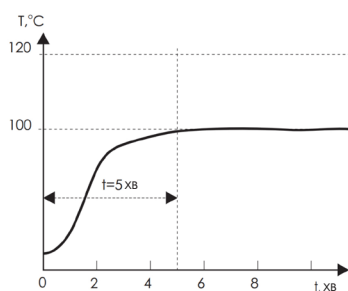
ПІД регулятор ПрАТ "ТЕРА" (налаштування, паяльник, T_z=100^\circ\text{C} )
