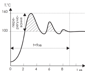
Стандартний ПІД регулятор (автоналаштування, паяльник, T_z=100^\circ\text{C} )
